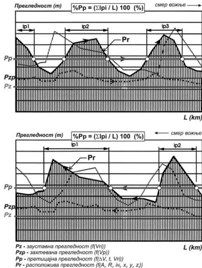
Слика 4-04: Профил расположиве прегледности.
