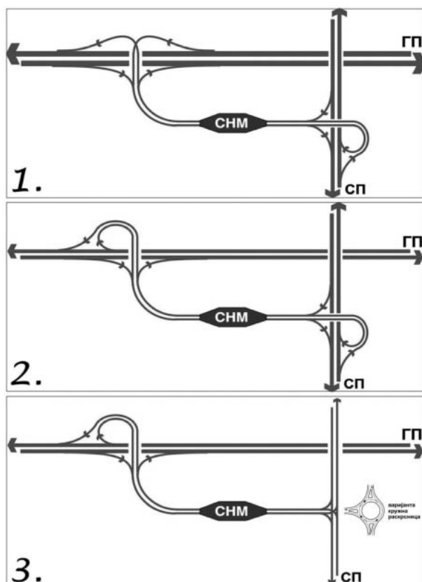
Слика 4-16: Типови денивелисаних раскрсница код комерцијалне експлоатације аутопутева: 1. Троугао-труба; 2. Дупла труба; 3. Индиректна труба.
