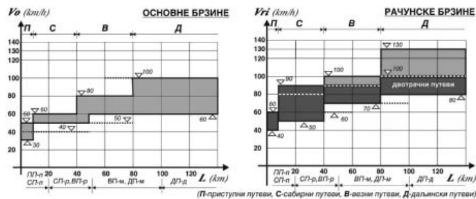
Слика 3-02: Приказ основне ( V_o ) и рачунске ( V_r ) брзине зависно од функционалне класификације ванградских путева и услова ограничења.
