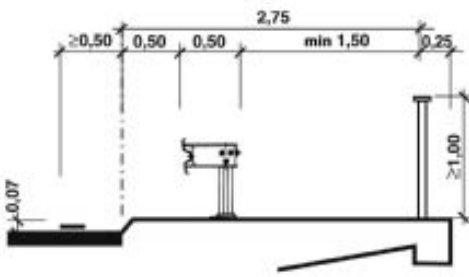
В) Пешачка стаза поред металне зашт. ограде
