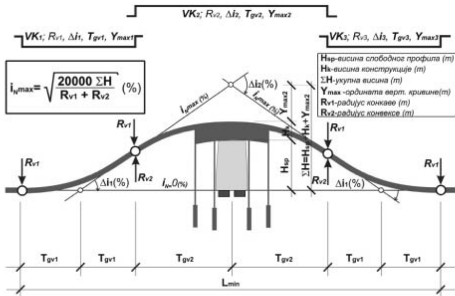
Слика 9-04: Геометријско одређивање минималних дужина навоза (max iN) када пут прелази преко сувоземних комуникација.
