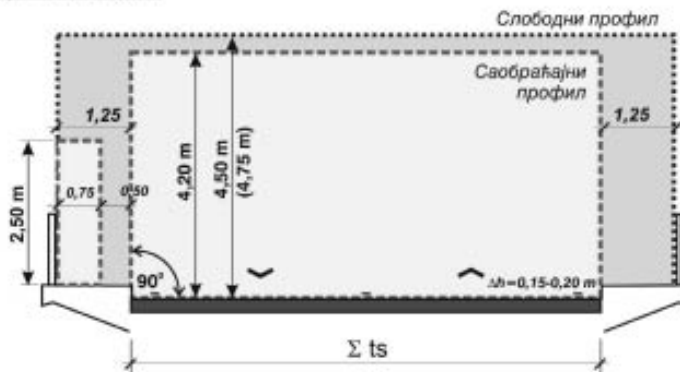
Слика 5-11: Слободни и саобраћајни профил двотрачног / вишетрачног пута.
