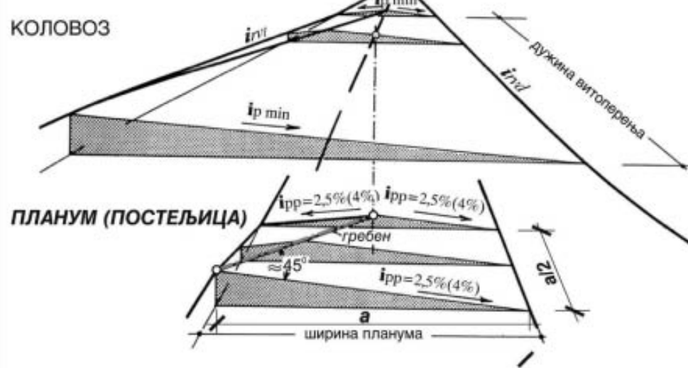
Слика 8-07: Витоперење плануа (постељице) пута.
