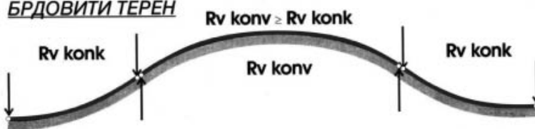
Слика 9-01: Основни просторни елементи трасе пута.
