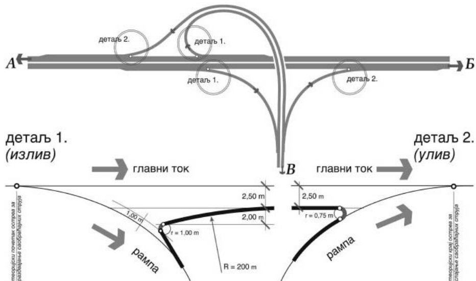
Слика 5-03: Обликовање завршетака острва на подручју излива и улива.
