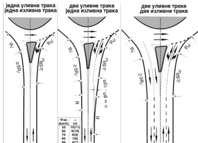
Слика 4-08: Типске конфигурације уливних и изливних трака кружне раскрснице (максимално усмеравање улива и излива).
