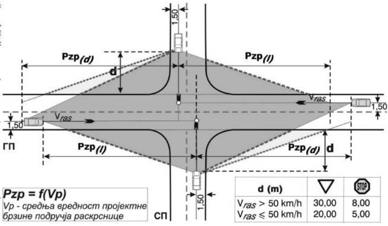
Слика 3-09: Конструкција зоне прегледности на четворокракој површинској раскрсници.
