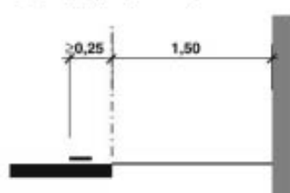
Слика 5-13: Радне, пешачке и бицикличке стазе на путним објектима.
