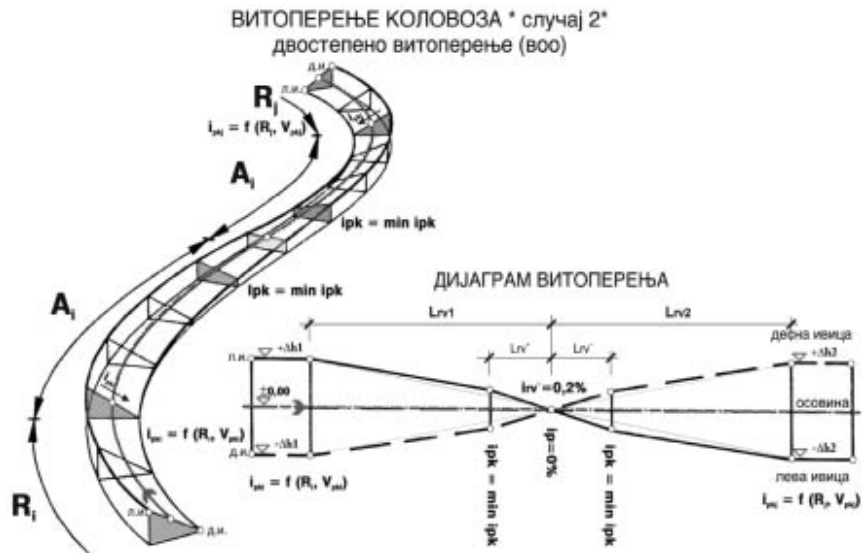
Слика 8-04: Двостепена промена попречног профила.
