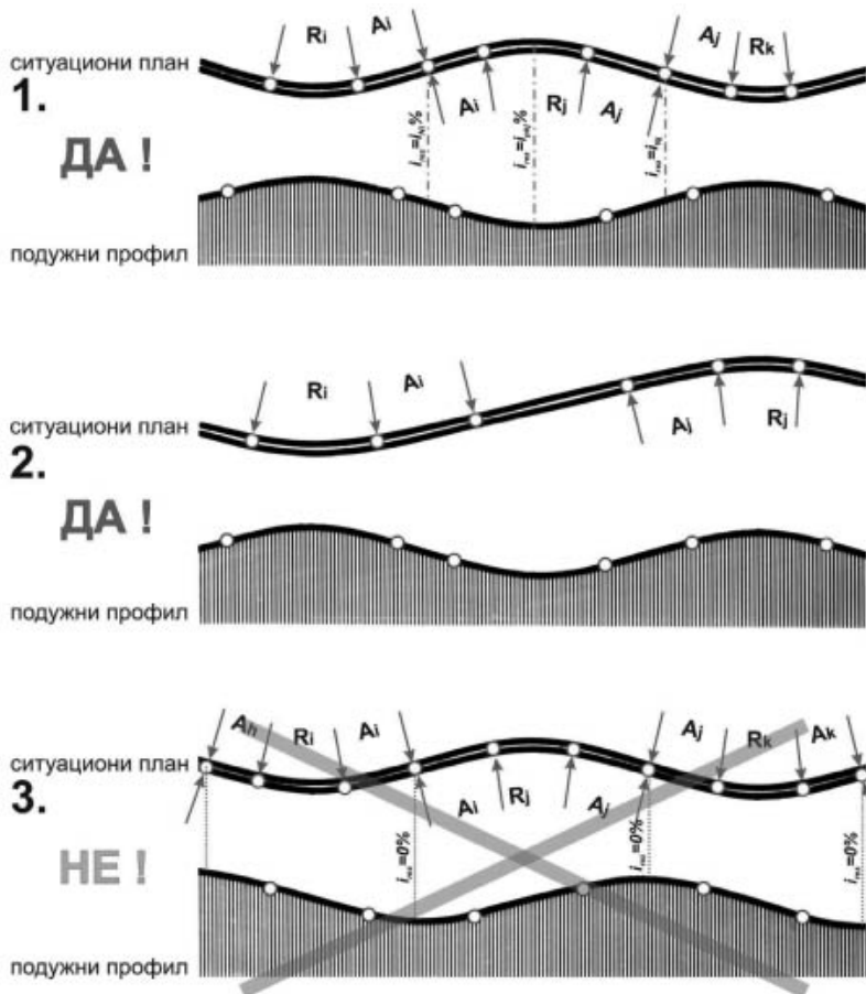
Слика 9-03: Просторно усклађење путних пројекција:
