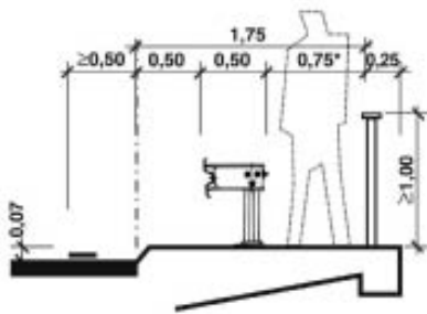
В) Пешачка стаза поред металне зашт. ограде
