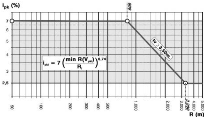
Слика 8-02: Номограм за одређивање величине попречног нагиба коловоза у кривинама (аутопутеви).
