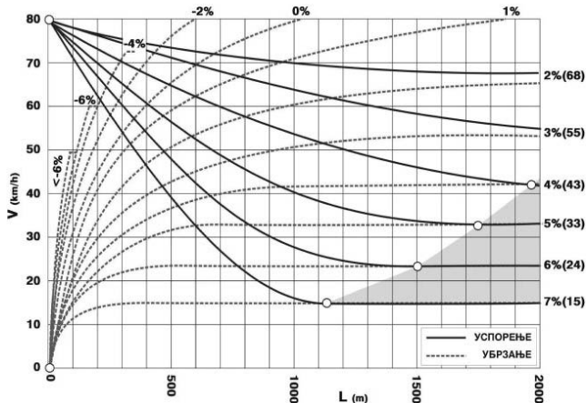
Слика 3-10: Дијаграм пута убрзања и успорења меродавног теретног возила.
