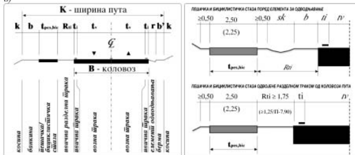
Слика 5-04: Карактеристични елементи геометријског попречног профила:
