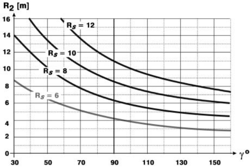
Слика 3-14: Избор полупречника кривине ( R_2 ) у зависности од скретног угла ( \gamma ) и меродавног возила: R_s = 6 - Путничко возило (ПА); R_s = 8 - Комби (ДВ); R_s = 10 - Камсион, Аутобус (ТВ, БУС); R_s = 12 - Ауто воз, Вучни воз (АВ, ВВ).
