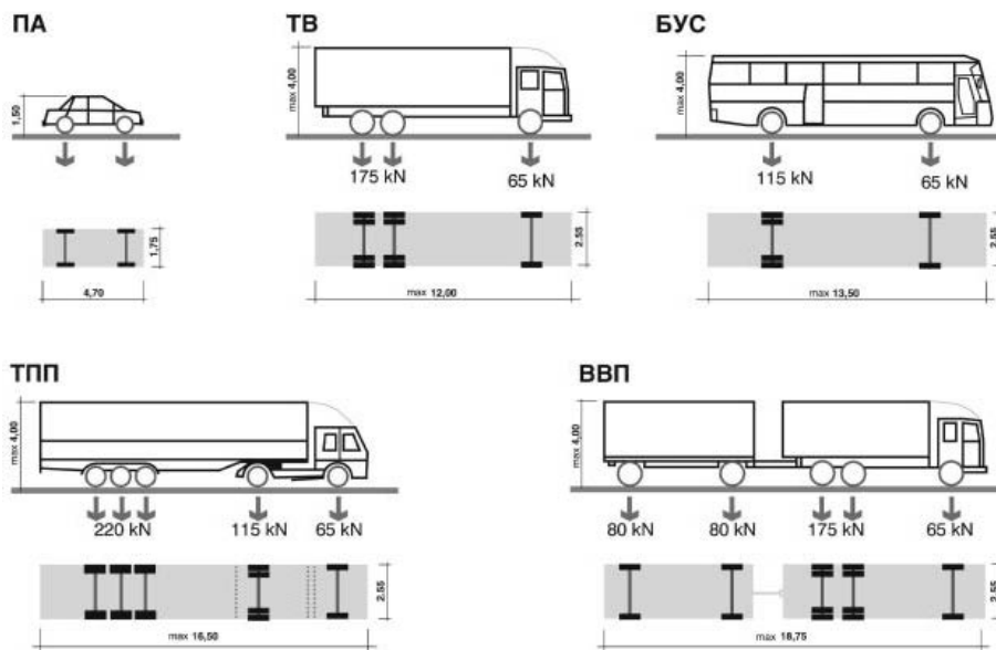
Слика 3-06: Карактеристичне габаритне мере меродавних возила.
