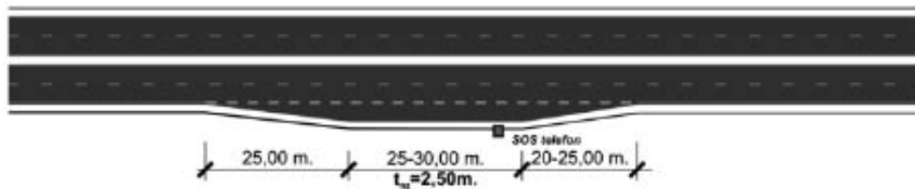
Слика 5-05: Стандардни облик нише за заустављање возила.
