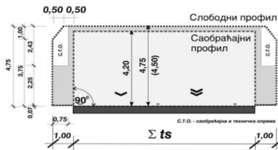
Слика 5-10: Слободни и саобраћајни профил аутопута у тунелу.
