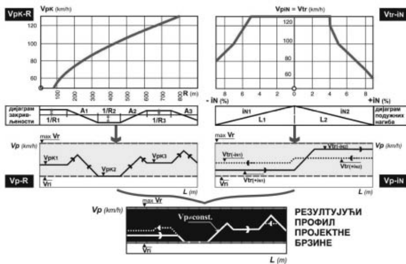
Слика 3-05: Конструкција резултујућег профила пројектне брзине.
