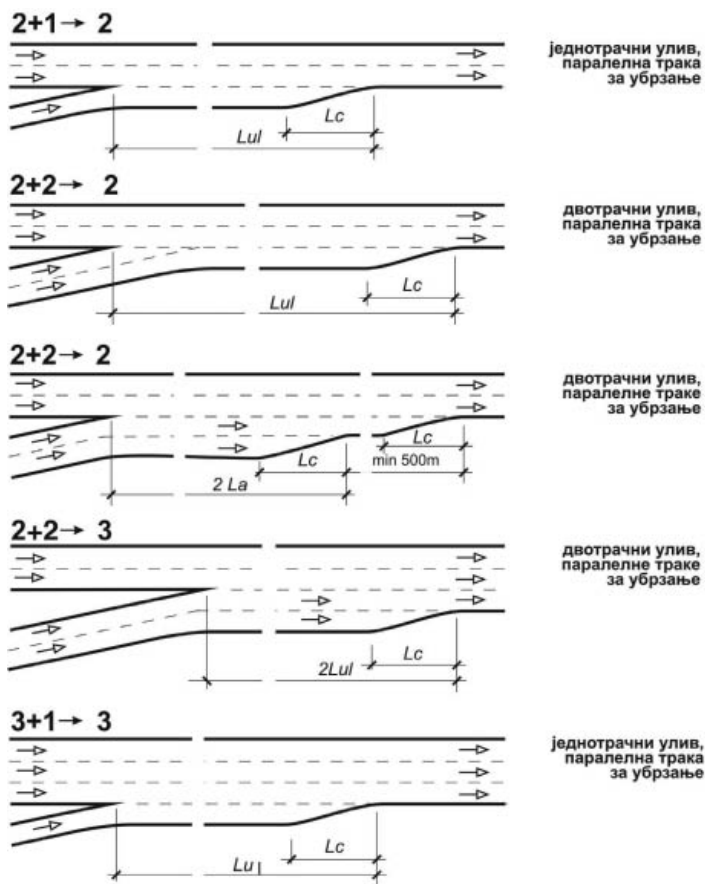
Слика 4-04: Типске конфигурације улива с могућим варијацијама броја возних трака.
