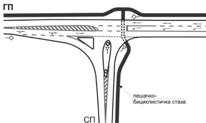
Слика 3-24: Пешачко-бицикличичка стаза у зони трокраке раскрснице.
