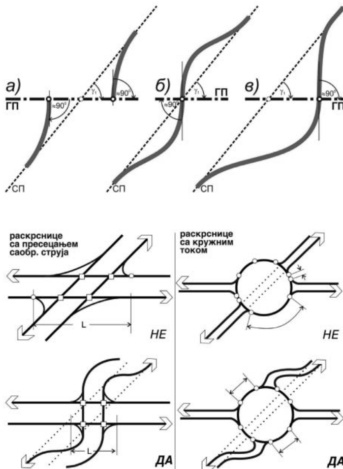
Слика 2-09: Примери лошег и исправног вођења споредног путног правца у зони раскрснице.
