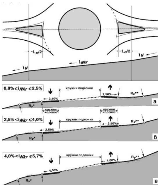
Слика 4-11: Ублажење подужних нагиба прикључних праваца на кружној раскрсници.
