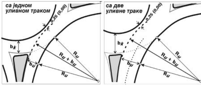
Слика 4-10: Почетни услов обликовања улива у кружни коловоз.
