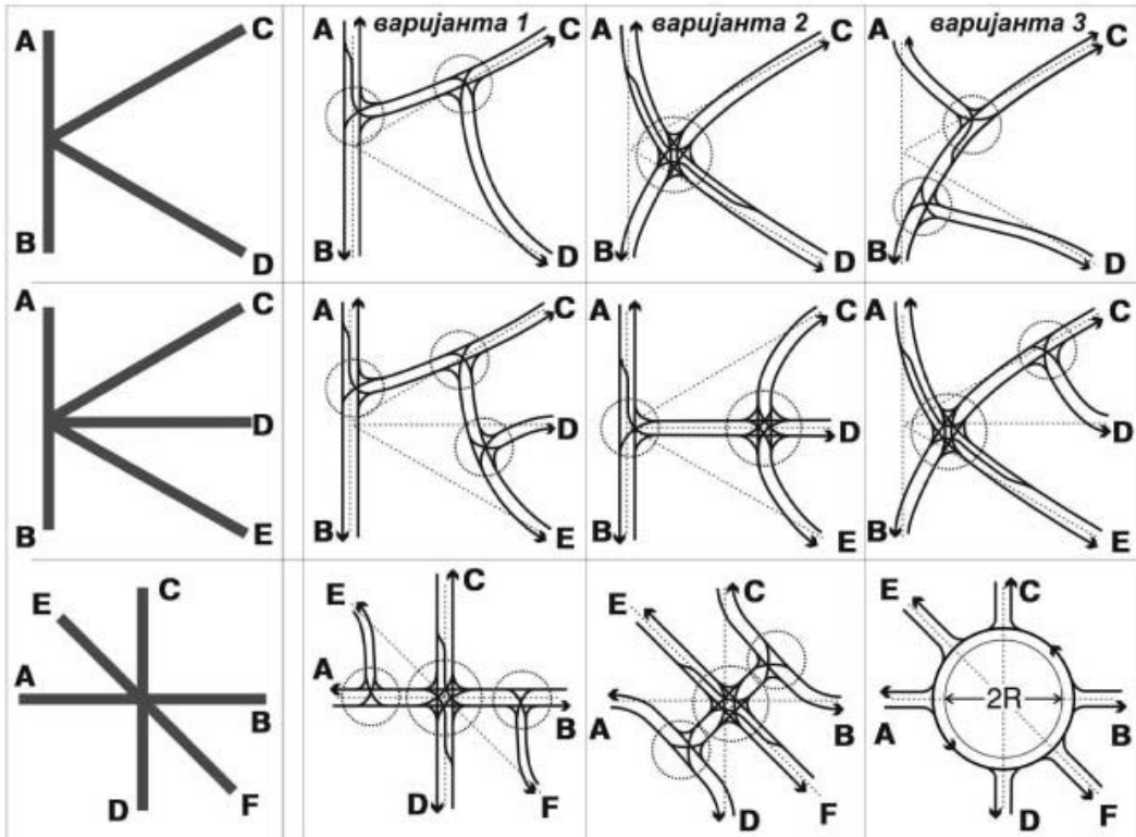
Слика 2-10: Примери просторног уређења (декомпозиције) пресечних (укрсних) праваца ради формирања типских површинских раскрсница.
